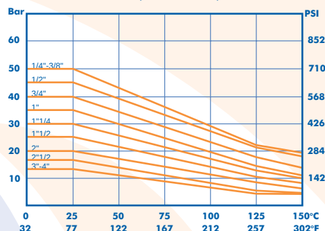
DIAGRAMA DE PRESION / TEMPERATURA / PASO COMPLETO
