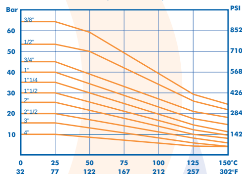
DIAGRAMA DE PRESION / TEMPERATURA / PASO REDUCIDO
