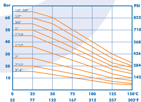
DIAGRAMA DE PRESION / TEMPERATURA
